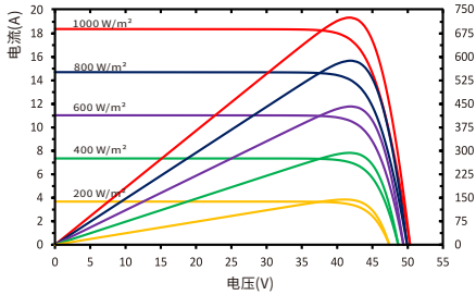
RSM132-8-730BHDG 不同辐照度下, I-V 曲线图
