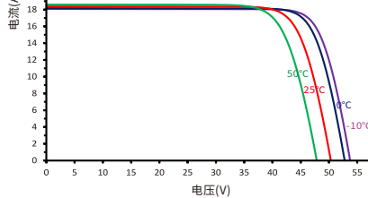
不同电池温度下, I-V 曲线图 (AM1.5, 1000W/m²)
